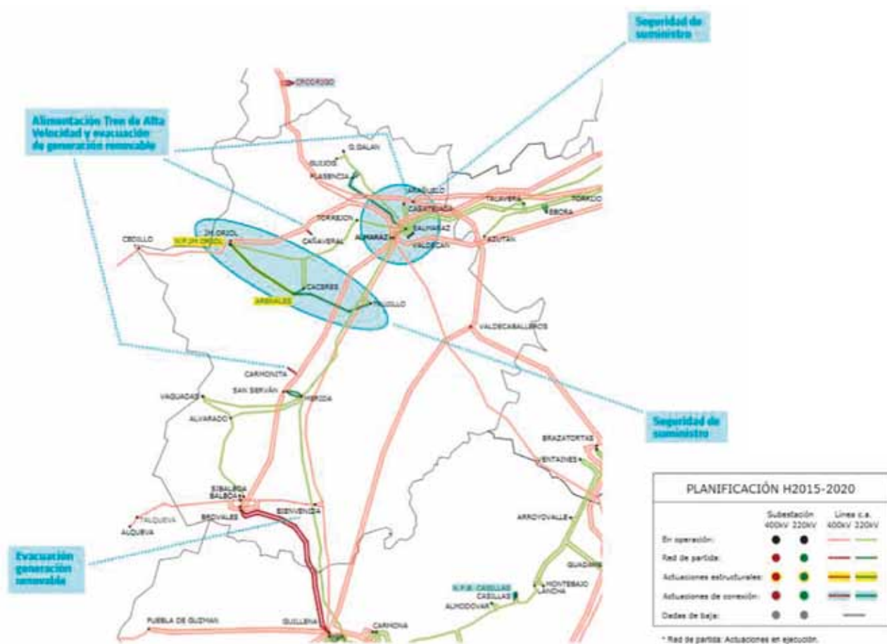
Imagen 10: Planificación de la red eléctrica extremeña para el periodo 2015-2020 (Fuente: REE)
